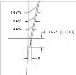
DOUBLE BEVEL
