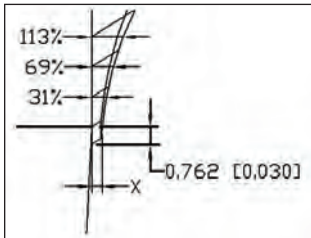
Double Bevel
