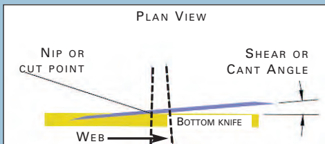
• Shear Angle
